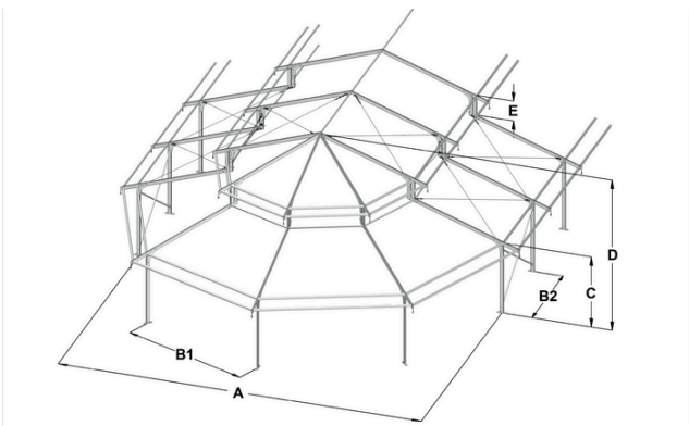
12m Levo Lite Apse
