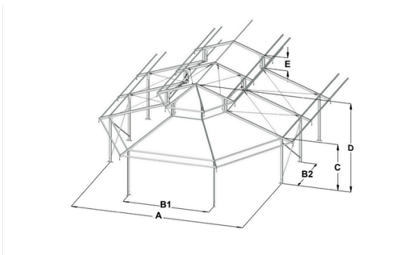
9m Levo Lite Apse
